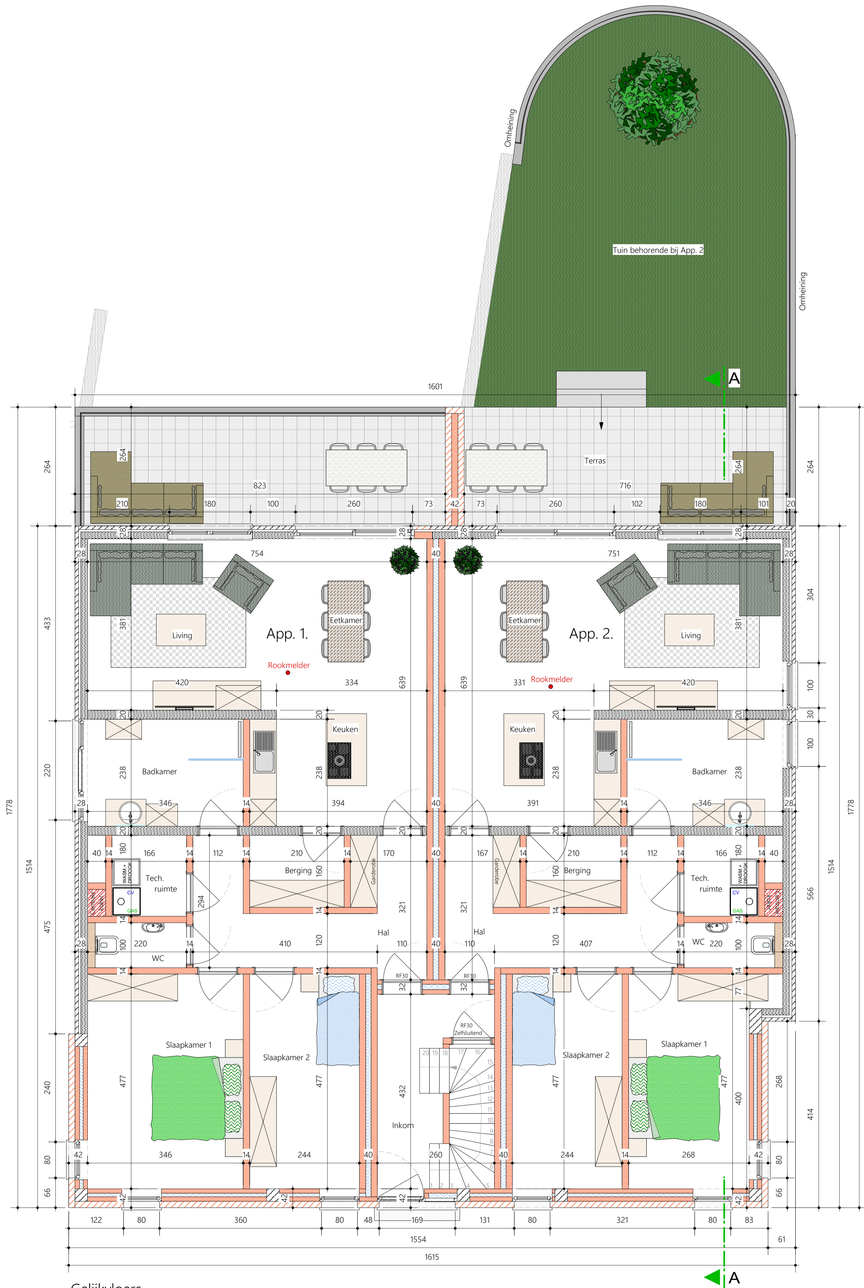
Gelijkvloers nieuwe toestand
